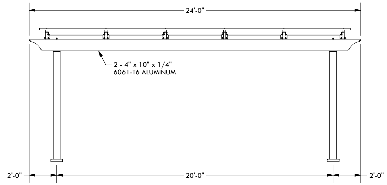
WIDTH ELEVATION
