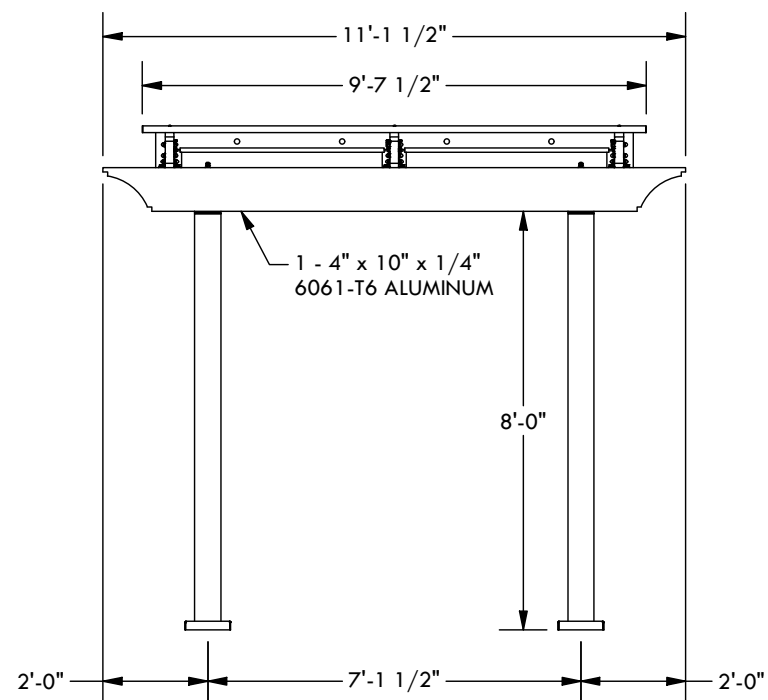
WIDTH ELEVATION
