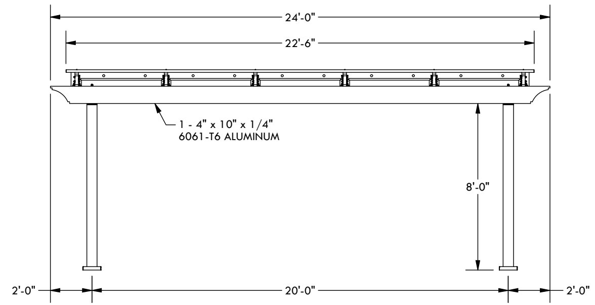
WIDTH ELEVATION
