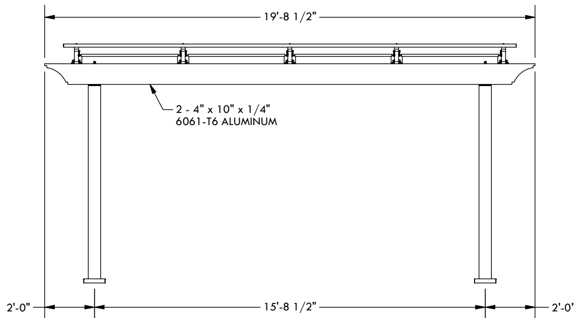
WIDTH ELEVATION
