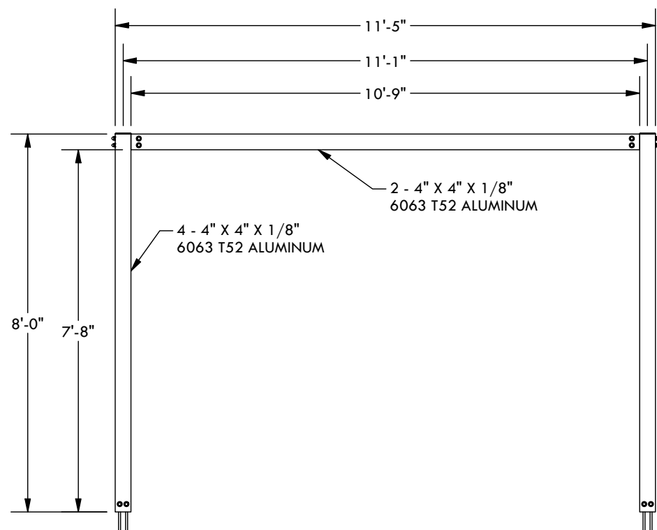
WIDTH ELEVATION
