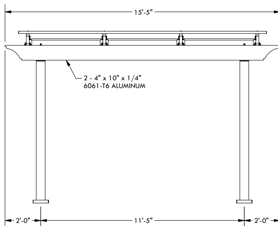
WIDTH ELEVATION
