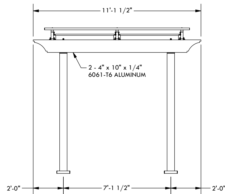
WIDTH ELEVATION
