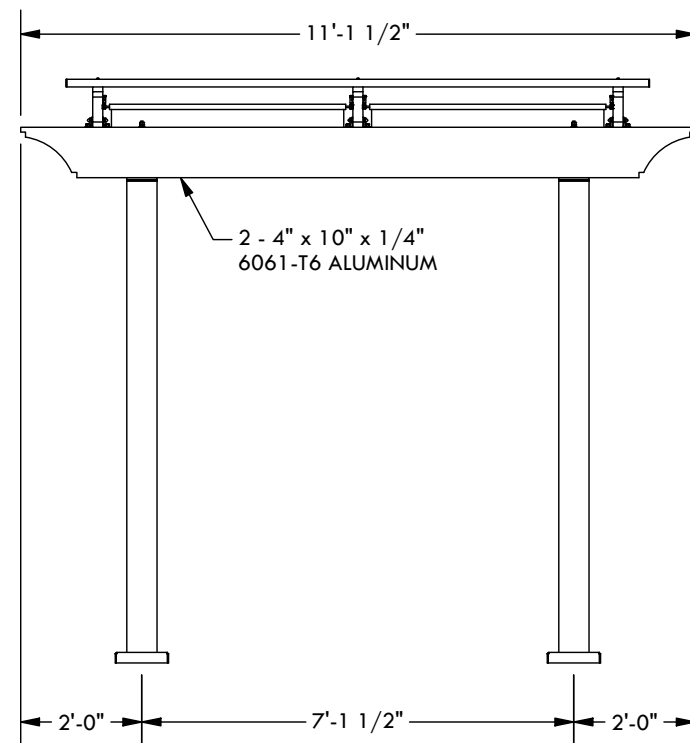
WIDTH ELEVATION
