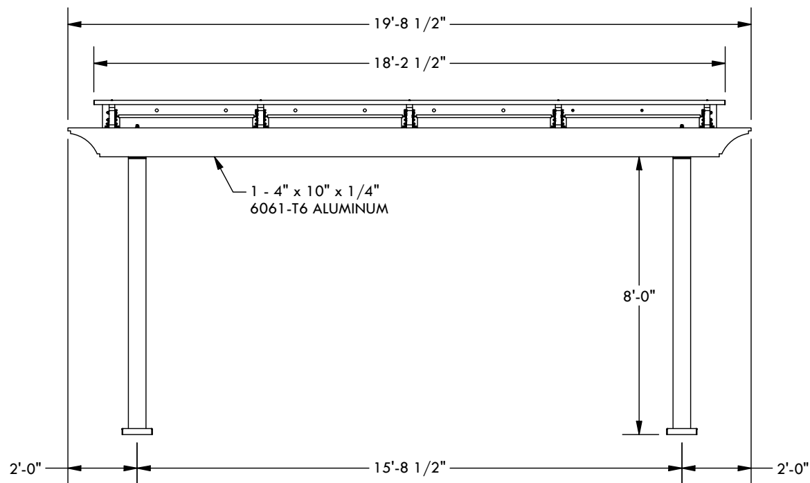
WIDTH ELEVATION
