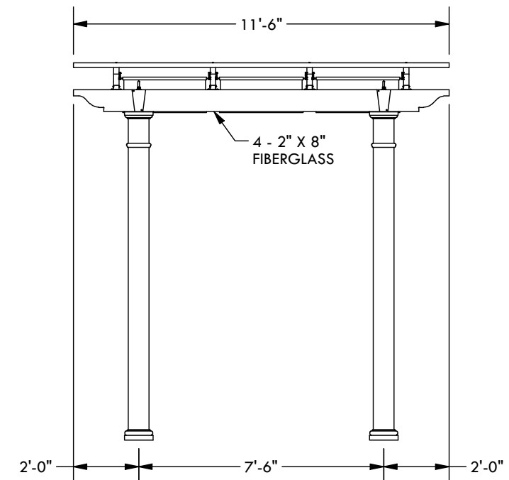
WIDTH ELEVATION
