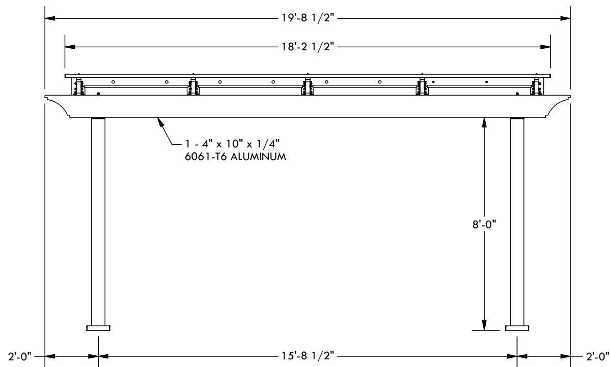
WIDTH ELEVATION
